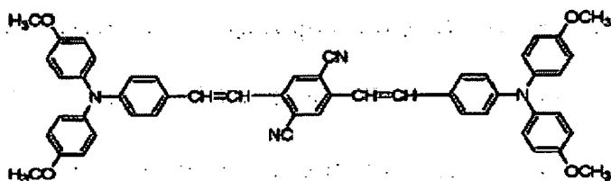
a-NPD:
